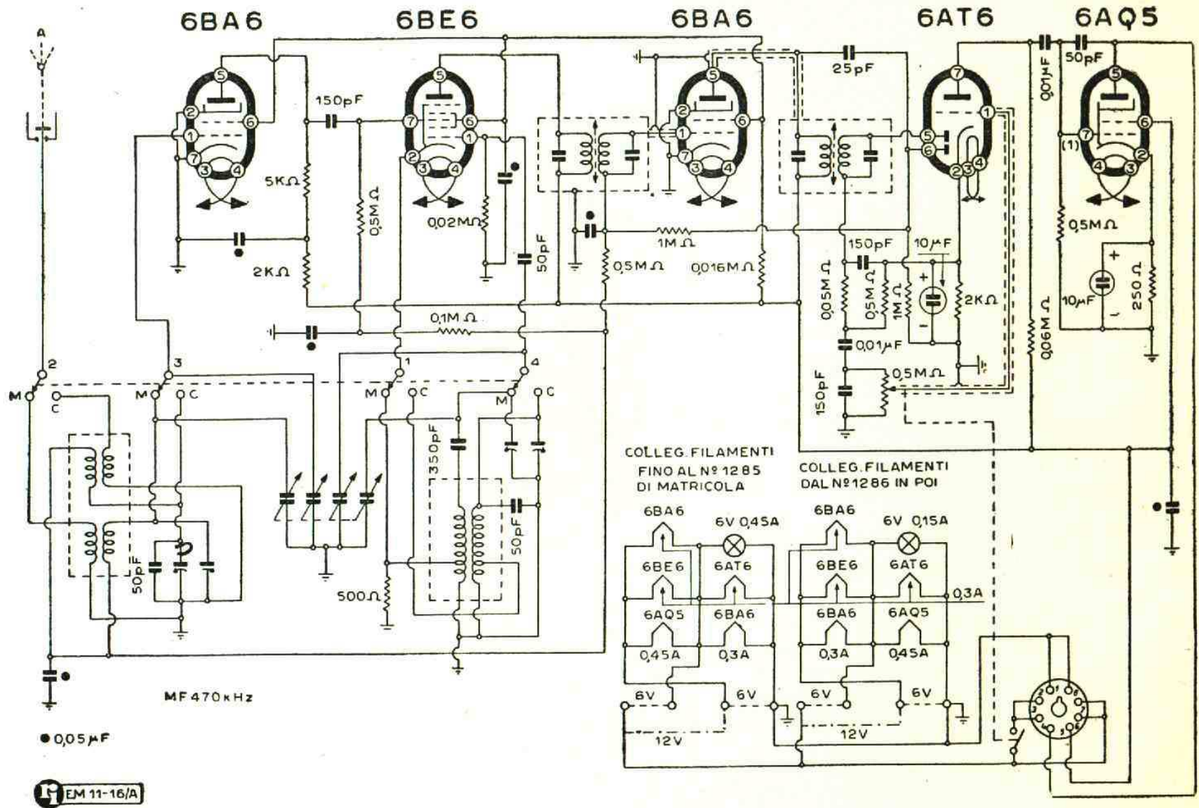
L'autoradio mod "Razzo,, (V. alimentazione nel verso).
